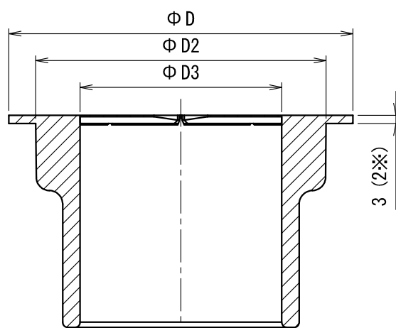
断面 A-A
